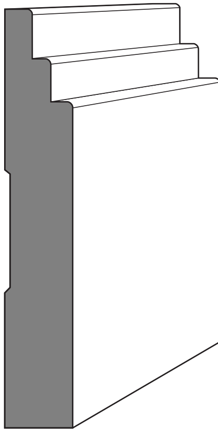
4 1/4" Step
