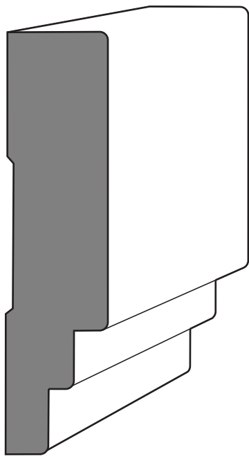
3 1/4" Step
